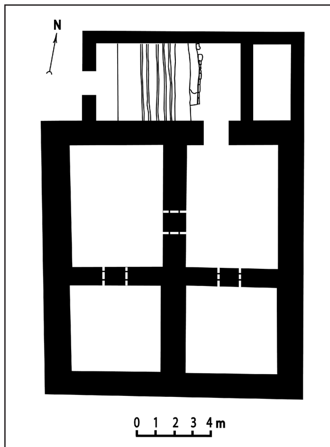
Рис. 1. План палацу І. Мазепи на передмісті Батурина Гончарівці (перед 1700 р.) за археологічними дослідженнями. Реконструкція
